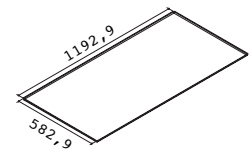
Bandeja Skin Modular para módulo de 610 x 1220
