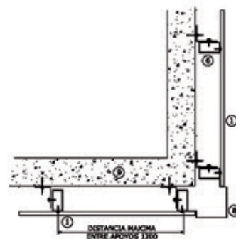
CORTE HORIZONTAL
